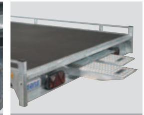
3 Aluminium Auffahrstufen integriert
