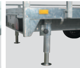
8 Kurbelstützen (Option)
